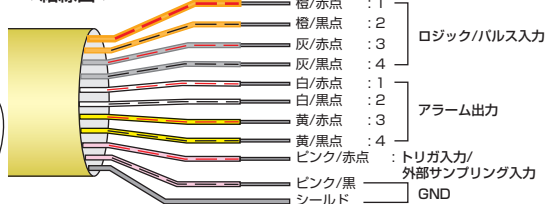
< 結線図 >
