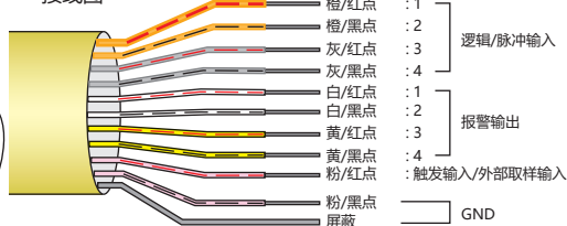
< 接线图 >
