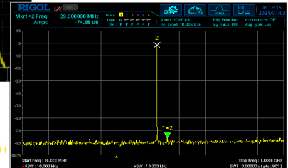
-70 dBc SFDR
